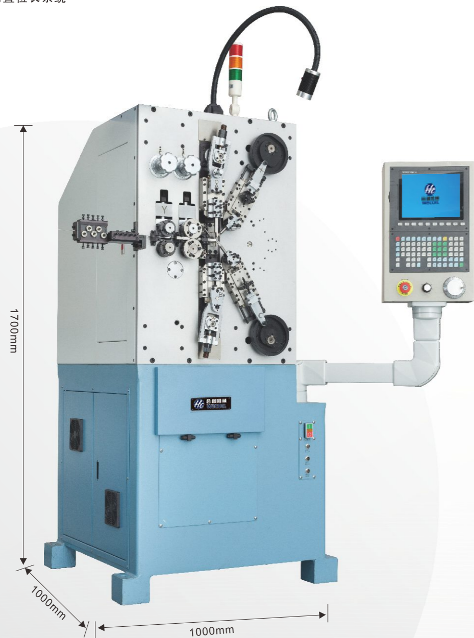
External/Internal spring length gauge 外置/内置检长系统
